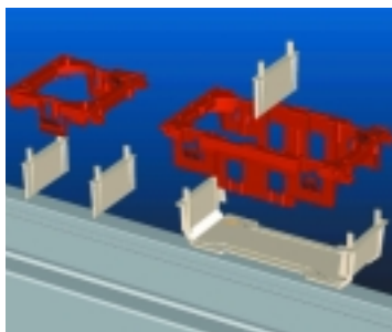
Skillevegg benyttes ved kombinasjonen sterk-/svakstrøm. Bunnplate med svekkinger kan leveres for å sikre isolasjon i metallkanaler.
