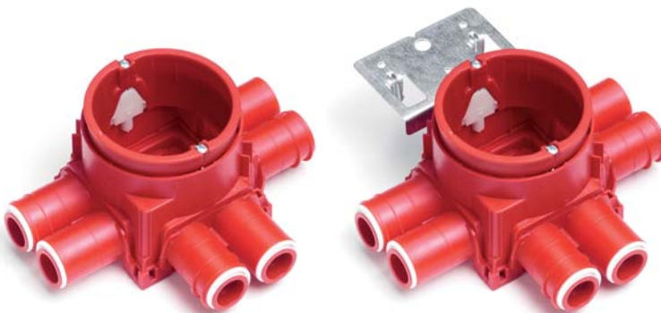
Flexi 20 veggboks høy ring for doble gipsplater.
