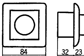
Målskisse
