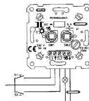
Koblingskjema
