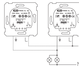
Koblings skjema
